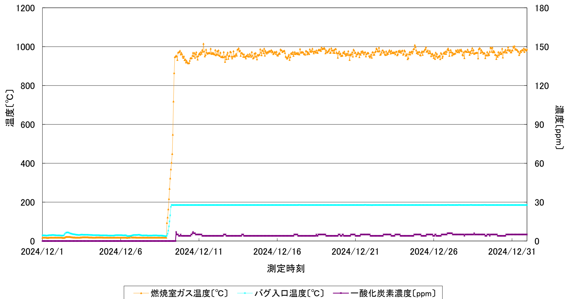
3号炉 連続測定結果 (燃烧室ガス温度、バグ入口ガス温度、一酸化炭素濃度)
