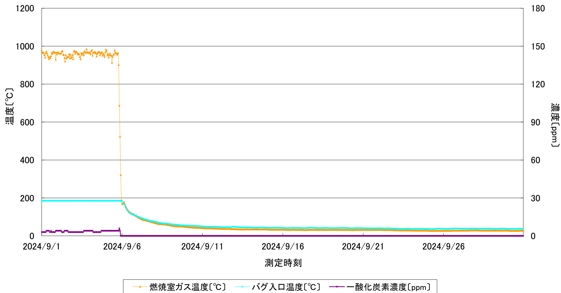
2号炉 連続測定結果 (燃焼室ガス温度、バグ入口ガス温度、一酸化炭素濃度)
