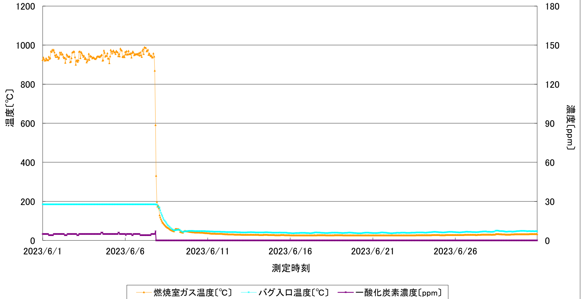
2号炉 連続測定結果 (燃烧室ガス温度、バグ入口ガス温度、一酸化炭素濃度)
