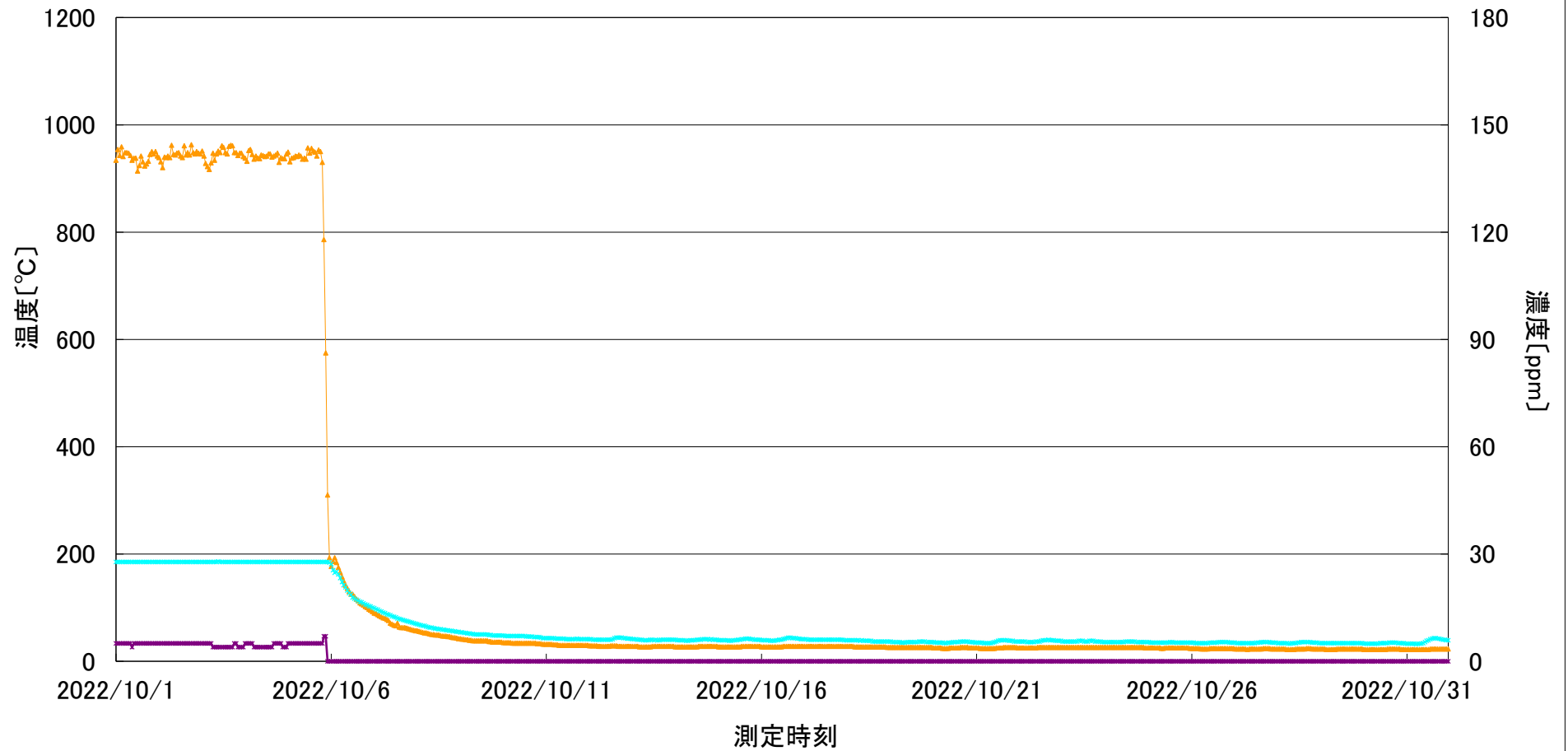
3号炉 連続測定結果 (燃烧室ガス温度、バグ入口ガス温度、一酸化炭素濃度)
