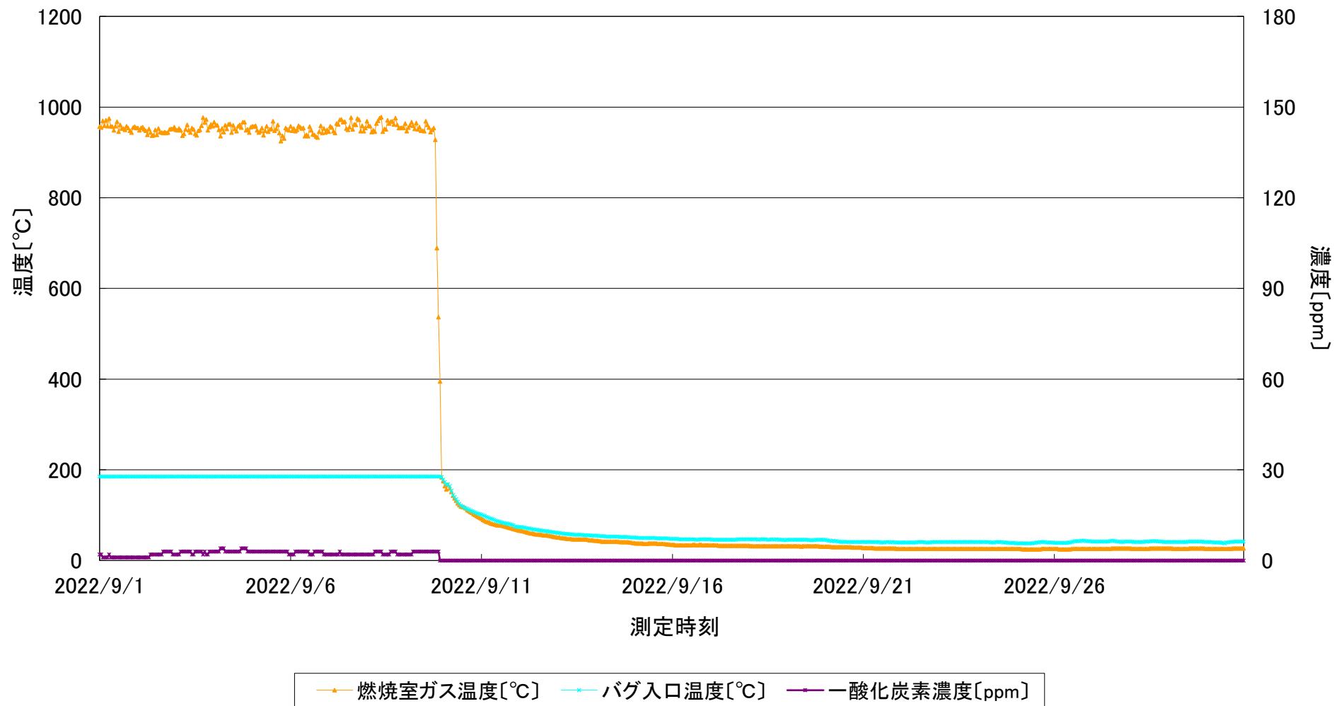
1号炉 連続測定結果 (燃烧室ガス温度、バグ入口ガス温度、一酸化炭素濃度)
