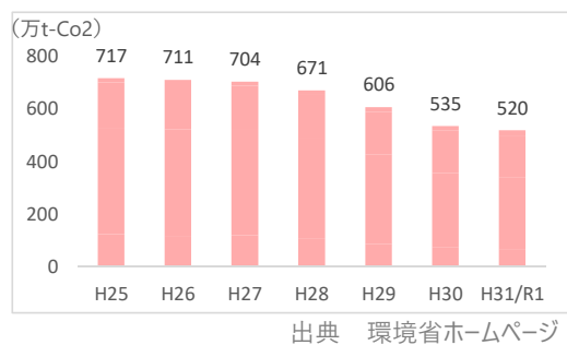
図10 市内の温室効果ガス排出量（推計）の推移
