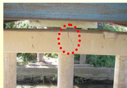
橋脚の損傷（ひびわれ）
